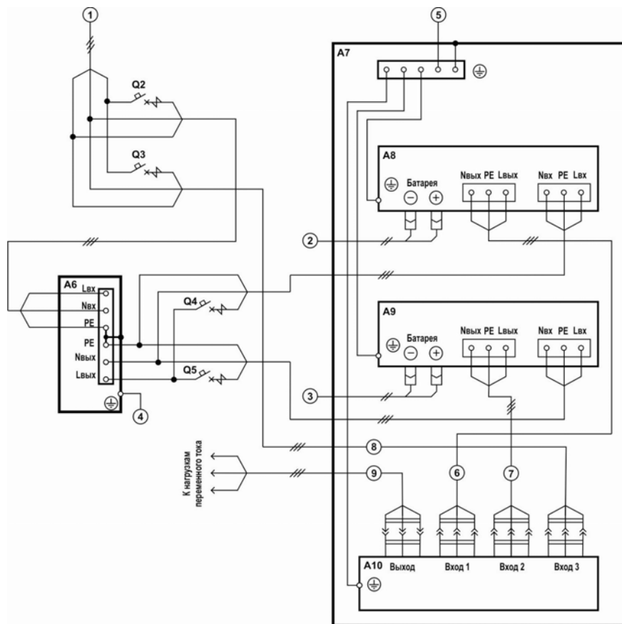
Рисунок Д.2 – Схема включения ПРП-1 по переменному току в составе СБЭП-48/325-12Б-С3 [окончание]
