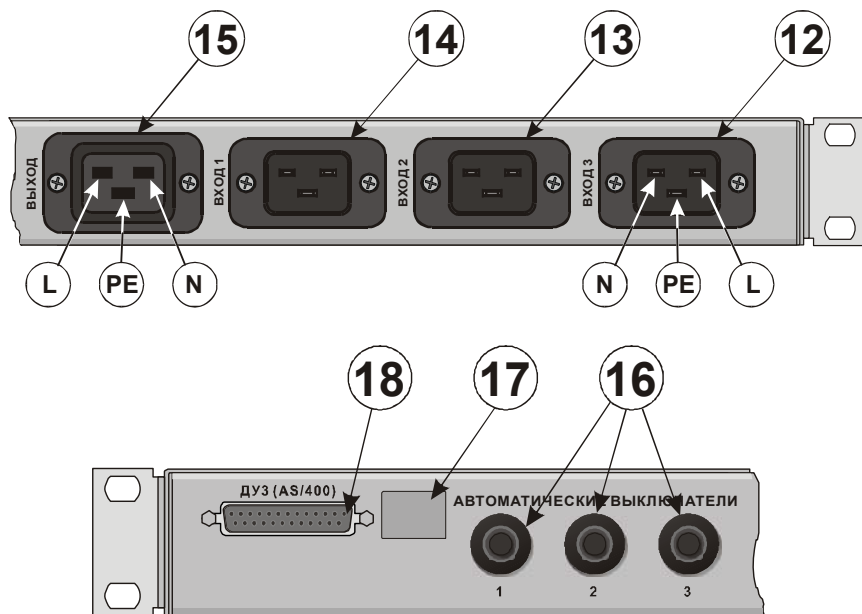
Рисунок 3 – Задняя панель ПРП
