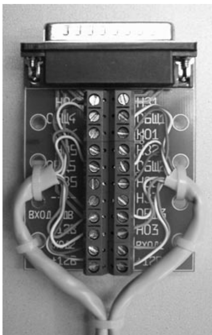
Рисунок 11 – Плата коммутационная КСДП.687253.020
