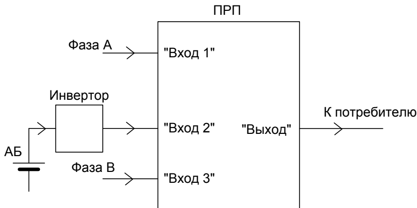
Рисунок 8 – Схема автоматической обводной цепи для инвертора или АБП
