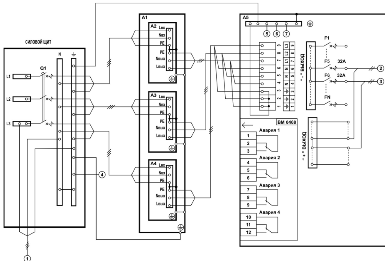
Рисунок Г.1 – Схема включения ПРП-1 по переменному току в составе СБЭП-48/160-6Б-С3 [начало]
