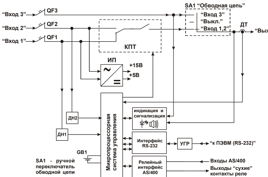
Рисунок 1 – Упрощенная структурная схема ПРП
