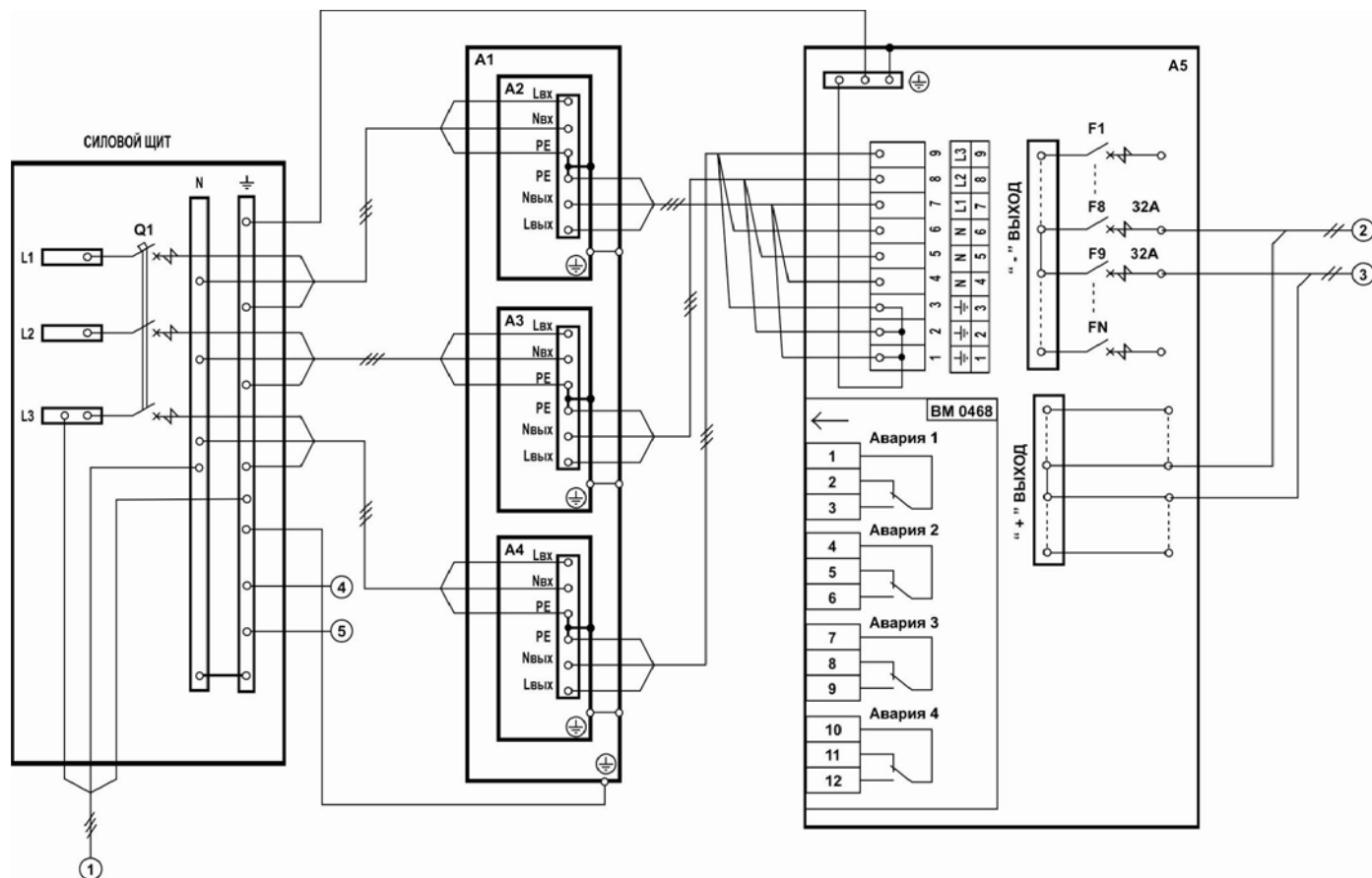
Рисунок Д.1 – Схема включения ПРП-1 по переменному току в составе СБЭП-48/325-12Б-С3 [начало]
