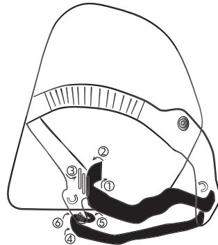
4. Вставить свободные концы резиновых лент в отверстия по аналогии с уже установленными
