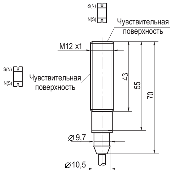
Габаритный чертеж
