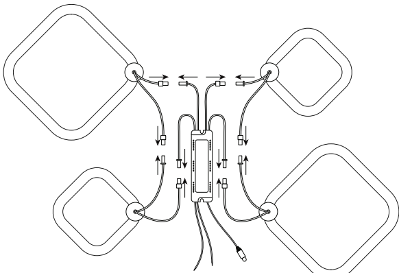
Схема подключения элементов плафона
