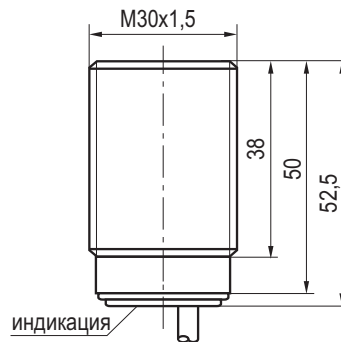
Габаритный чертеж
