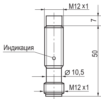
Габаритный чертеж
