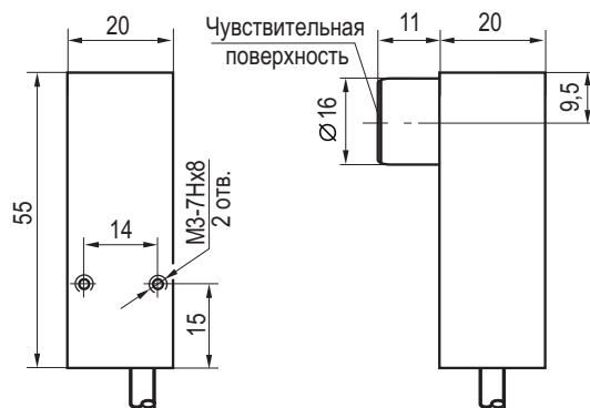
Габаритный чертеж
