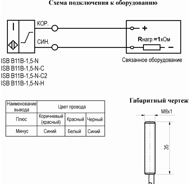
Схема подключения к оборудованию
