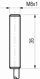
Габаритный чертеж
