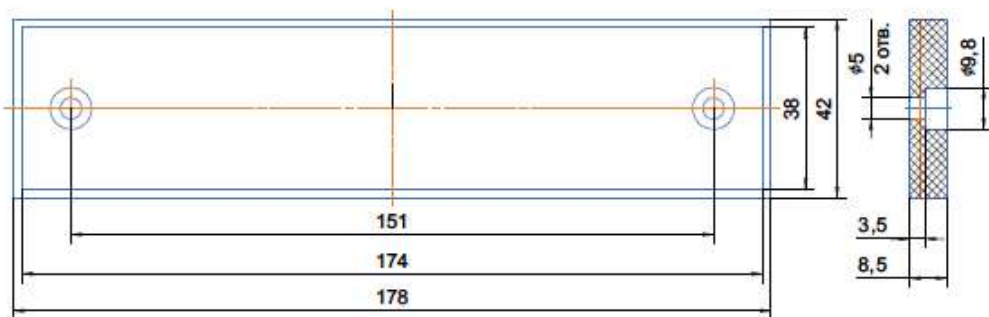
Габаритный чертеж
