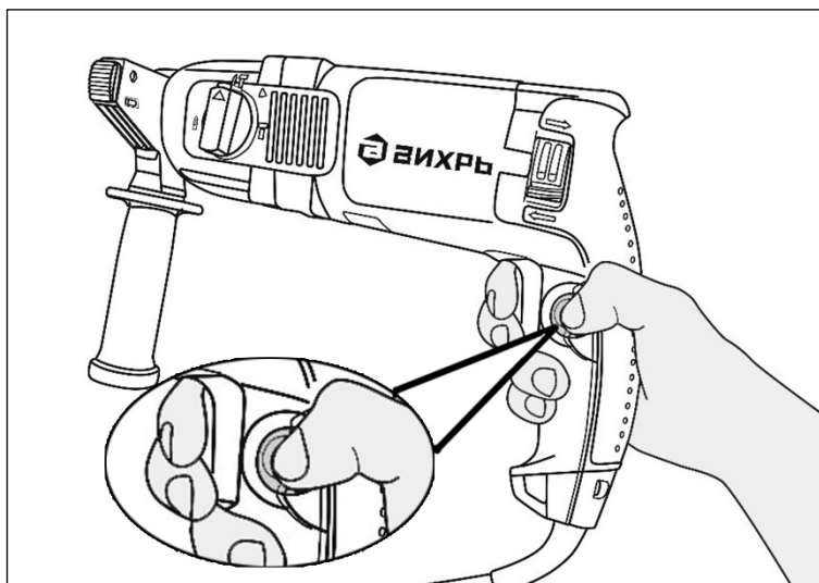
Рис. 11. Нажатие кнопки фиксации включателя
