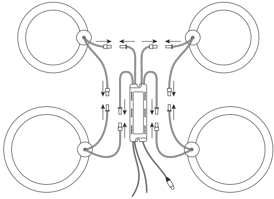
Схема подключения элементов плафона
