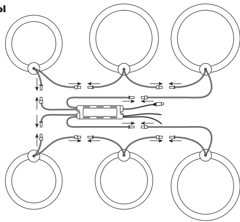
Схема подключения элементов плафона
