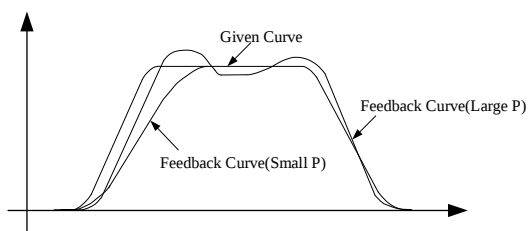
Рис. 8 Эффект отслеживания обратной связи от пропорциональной константы P
