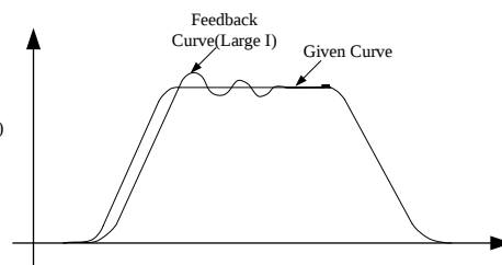
Рис. 9 Эффект отслеживания обратной связи от пропорциональной константы I
