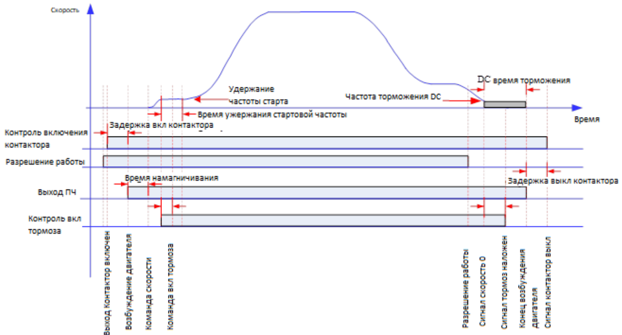
Рис. Диаграмма регулируемой временной последовательности (P00.02=5)
