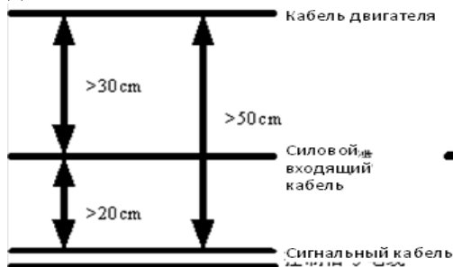
Рис2.(а) Параллельная прокладка
