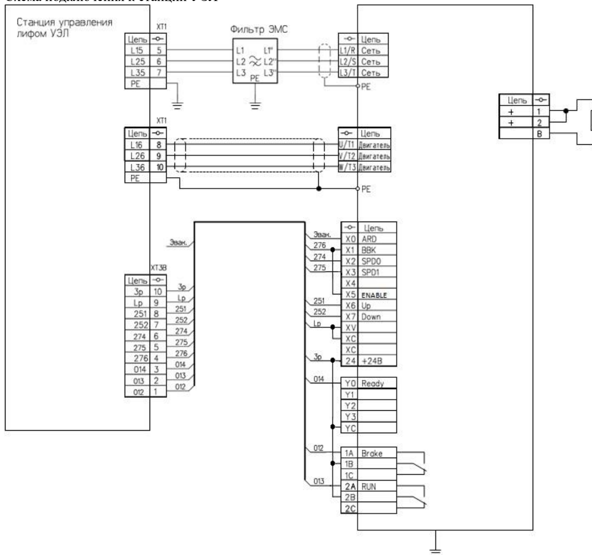
Рис. 36 Подключение ПЧ AS 620/AS320 к станции УЭЛ
