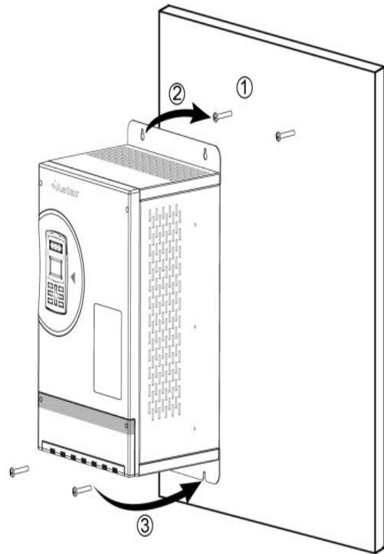
Рис.1б. Установка на панель
