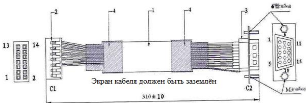
Рисунок 4 – Разъём для подключения энкодера
