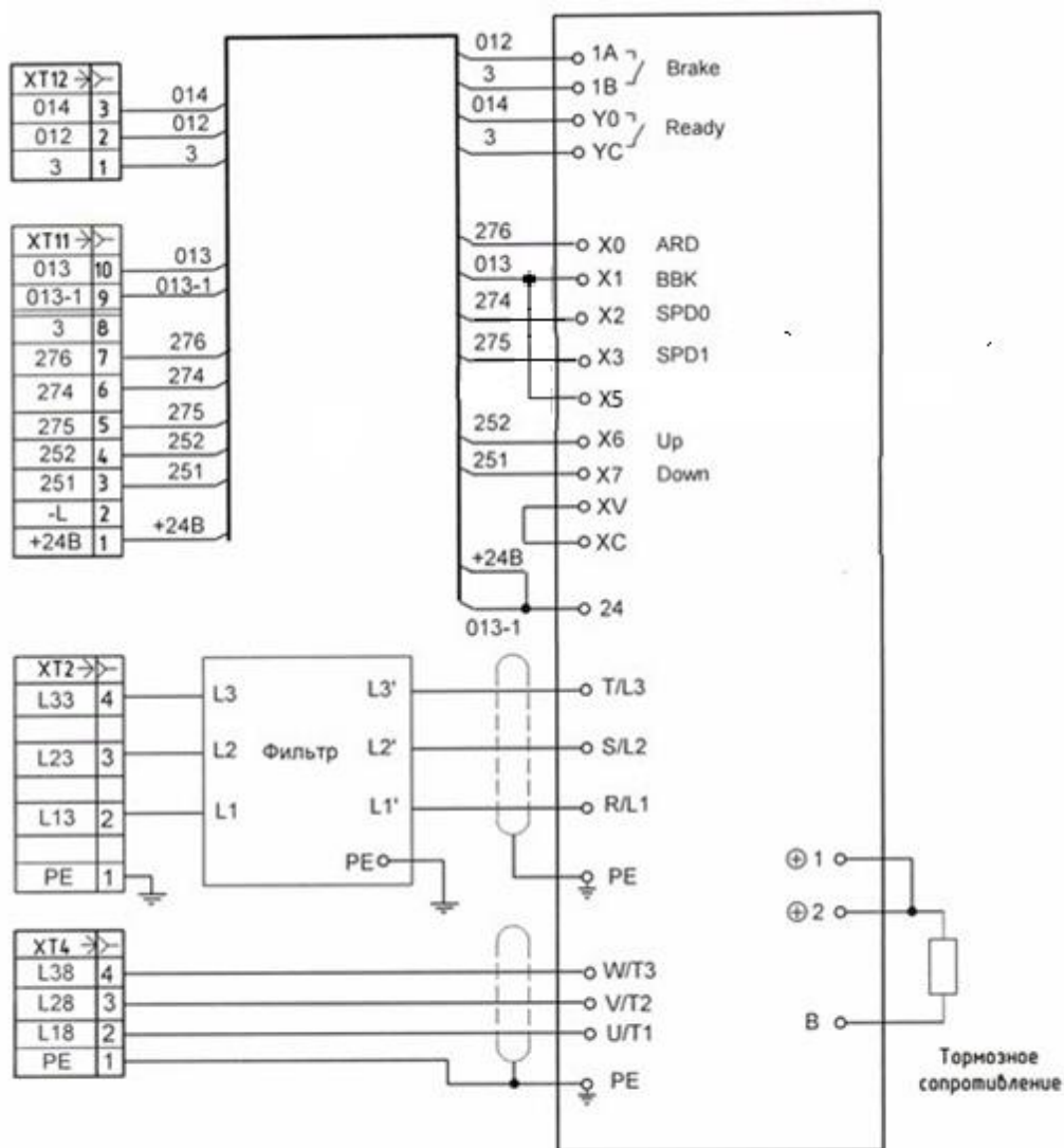
Рис.3а Подключение ПЧ AS 620/AS320 к станции управления ШК6000
