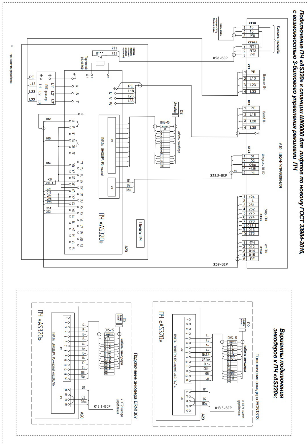
Рис.36 Подключение ПЧ AS320 к станции управления ШК6000- 3 бита скорости
