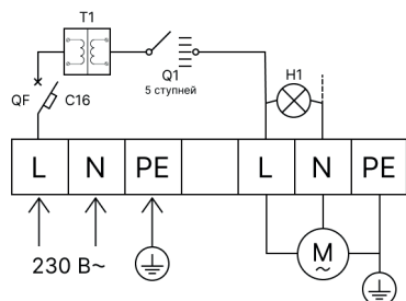
Схема подключения
