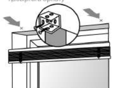
1C Установка сбоку оконного проема Терезе ойығының бүйірін орнату
