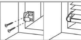
Установка прижимных кронштейнов Қысу кронштейндерін орнату
