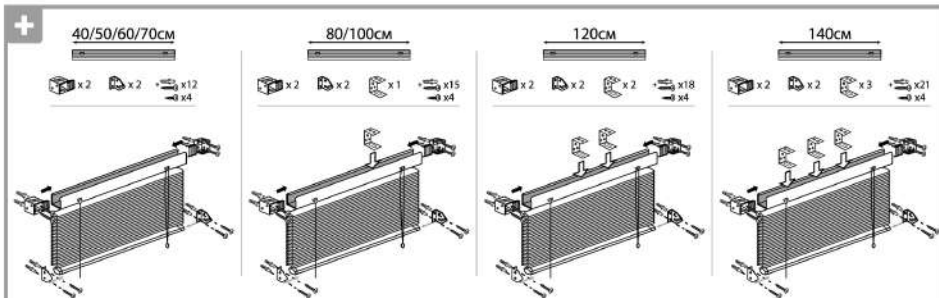
1A Установка сверху оконного проема Терезе ойығының үстіне орнату
