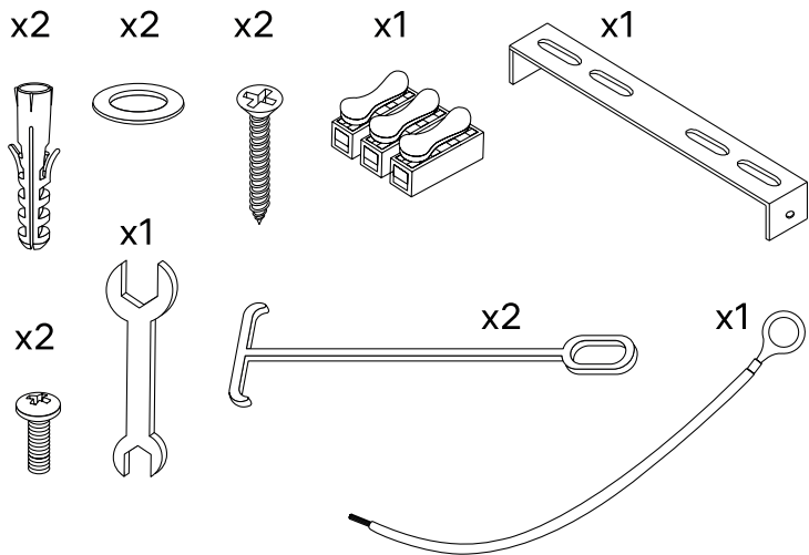
2. Монтажный комплект
