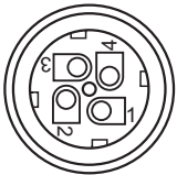
Цоколевка соединителя (вид со стороны монтажа)
