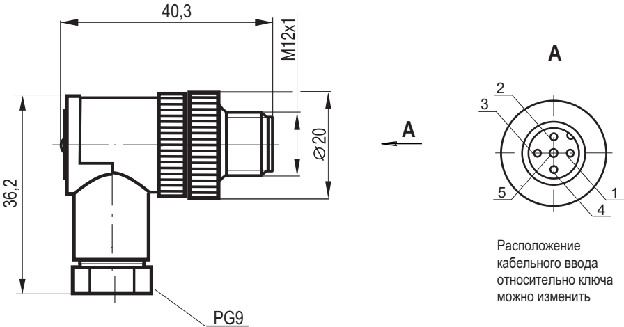
Габаритный чертеж
