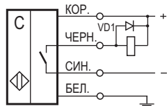
Схема подключения индуктивной нагрузки (реле)
