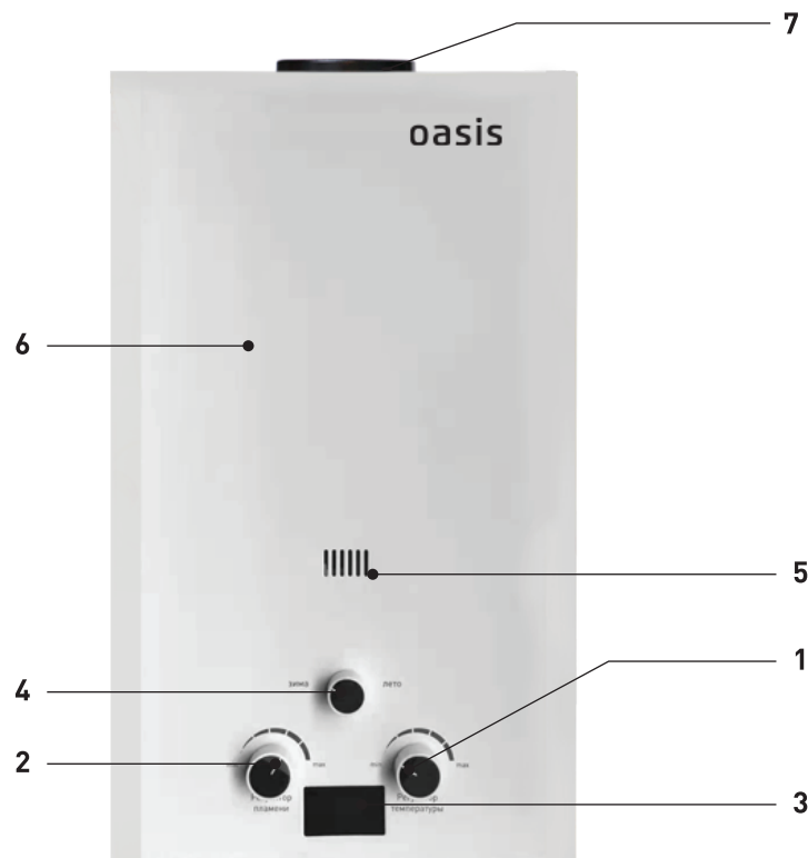
Рис. 1. Аппарат водонагревательный проточный газовый бытовой OASIS 1 - ручка водяного регулятора; 2 - ручка газового регулятора; 3 - цифровой индикатор температуры горячей воды; 4 - переключатель зима/лето; 5 - окно смотровое; 6 - облицовка; 7 - патрубок дымоотвода.
