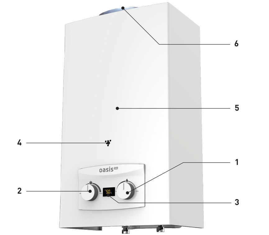
Рис. 1. Аппарат водонагревательный проточный газовый бытовой oasis pro 1 - ручка водяного регулятора; 2 - ручка газового регулятора; 3 - цифровой индикатор температуры горячей воды; 4 - окно смотровое; 5 - облицовка; 6 - патрубок дымоотвода.
