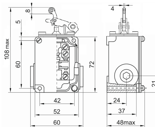
Рис.4. ВПК 2113 БУ2 – привод селективный
