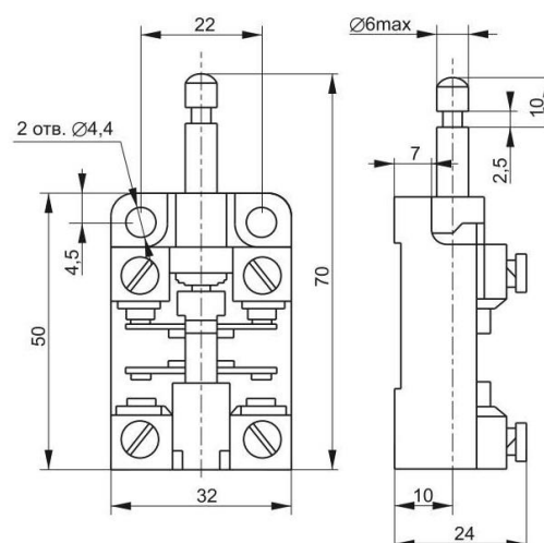
Рис.6. ВПК 2010 БУХЛ4 Д/Т
