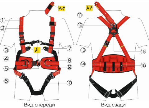
Страховочная привязь модель ST5 (арт. STR103)
