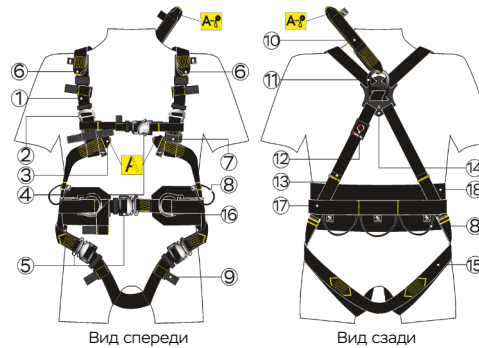
Страховочная привязь модель ST5N (арт. STR103N)
