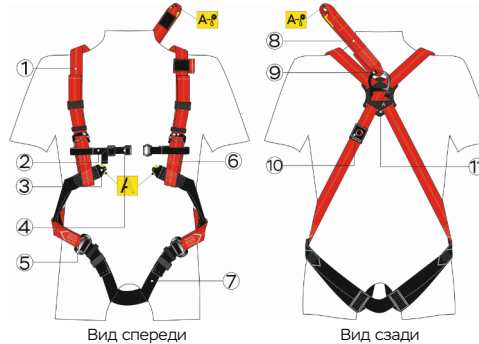
Страховочная привязь модель ST3 (арт. STR003)
