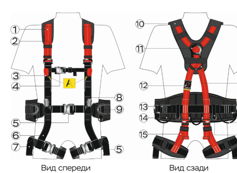
Страховочная привязь модель CANYON (арт. STR110)
