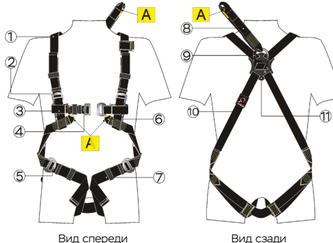
Страховочная привязь модель ST3N (арт. STR003N)
