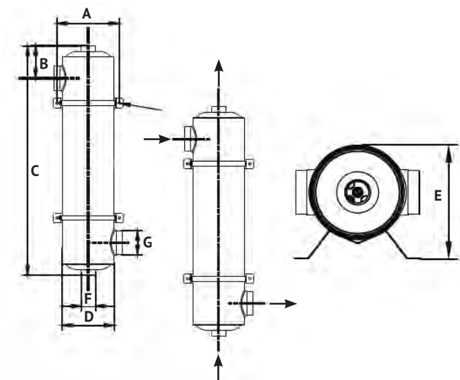
Рисунок 1 – Габаритные и присоединительные размеры
