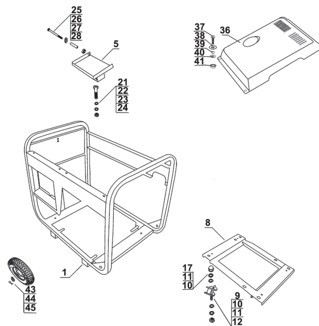
Схема сборки № 5
