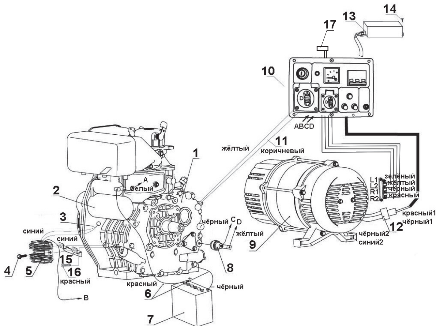
Схема сборки № 1
