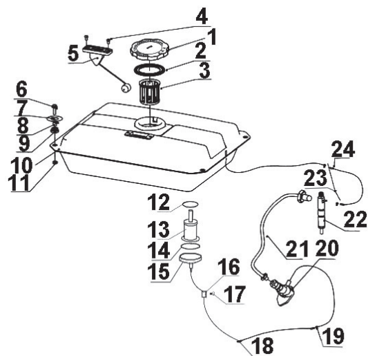
Схема сборки № 4
