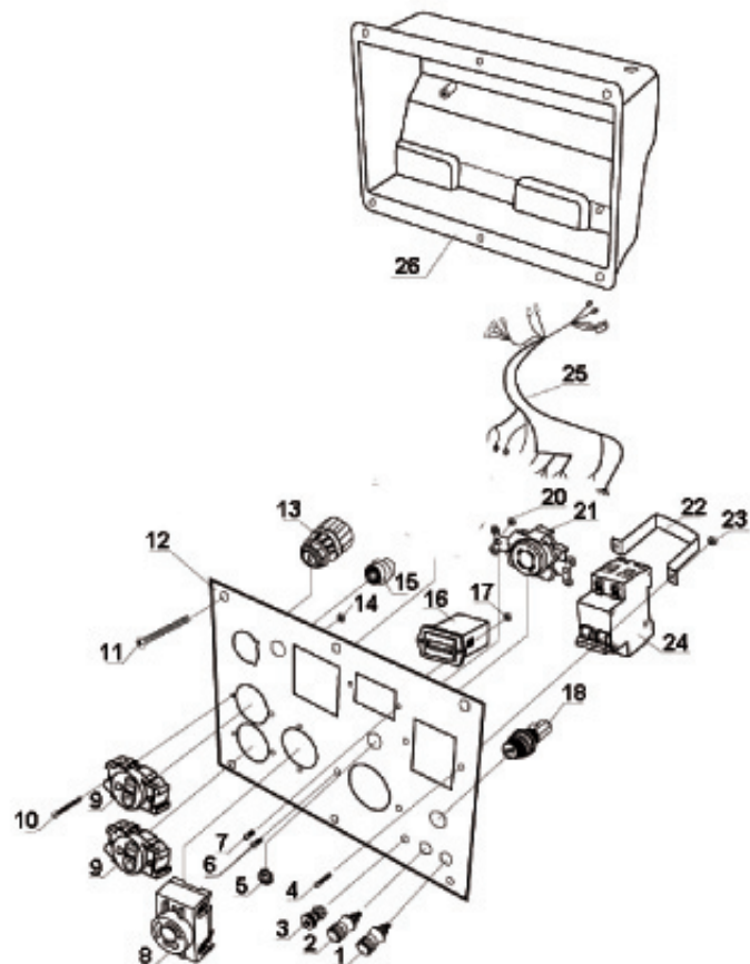
Схема сборки № 2
