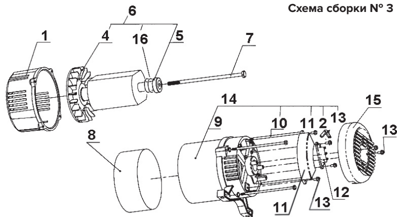
Схема сборки № 3
