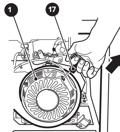
17. Рукоятка
