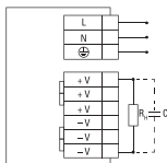
Рис 8. Схема подключения (MPS-200W-12, MPS-350W-12)
