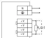
Рис 7. Схема подключения (MPS-100W-12, MPS-150W-12)
