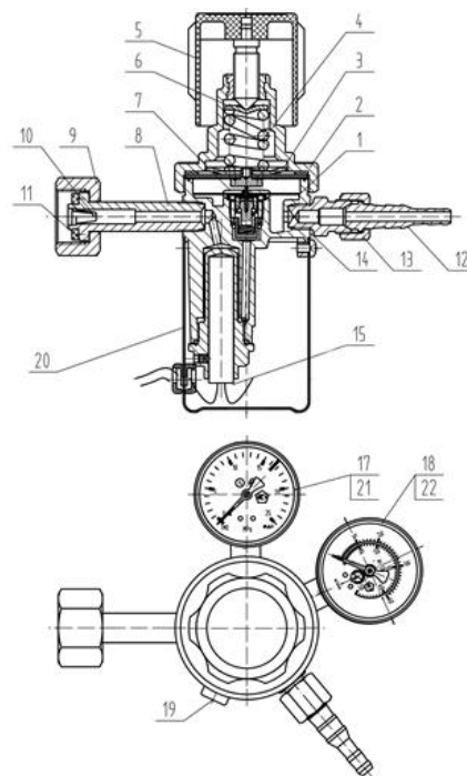
Рис. 4. Регулятор расхода газа баллонный одноступенчатый У 30 KPP:
