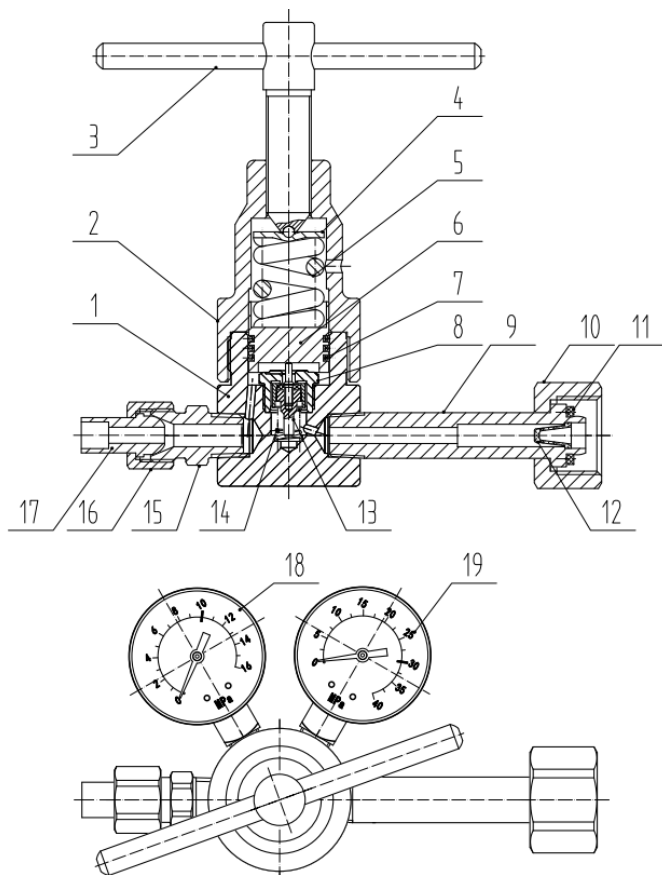
Рис. 1. Редуктор баллонный одноступенчатый.
