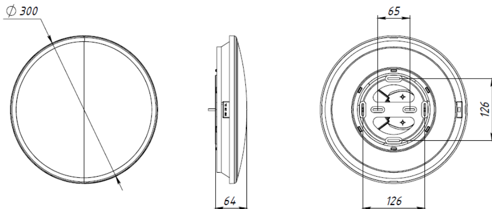
Рисунок 1. Габаритные размеры светодиодного светильника Orbita Smart 24Вт.
