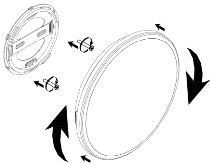
Рисунок 3. Монтаж светильника на поверхности.
