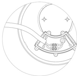
Рисунок 2. Подключение светильника.
