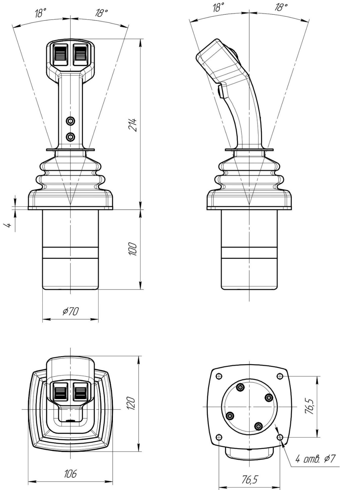
Рисунок 2. Габаритно – присоединительные размеры.
