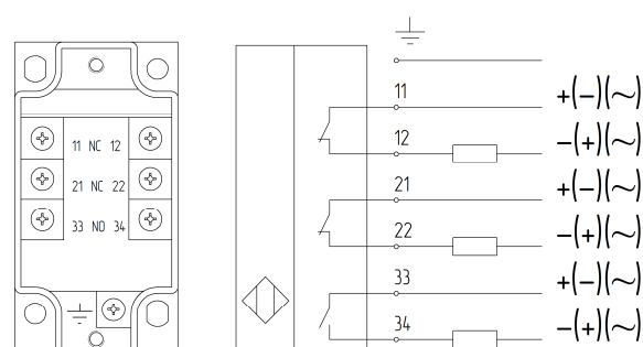
Рисунок В2: Расположение клемм и схема подключения, 2 вариант
