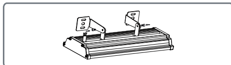
4. Монтаж при помощи подвесов
