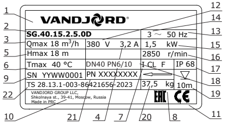
Рис. 2 Фирменная табличка
