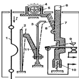
1-сурет. Жылулық жүктеме релелерінің құрылымдық схемасы.
