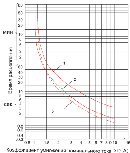
Рисунок 2. Время-токовая характеристика реле теплового перегрузки серии РТ-02
