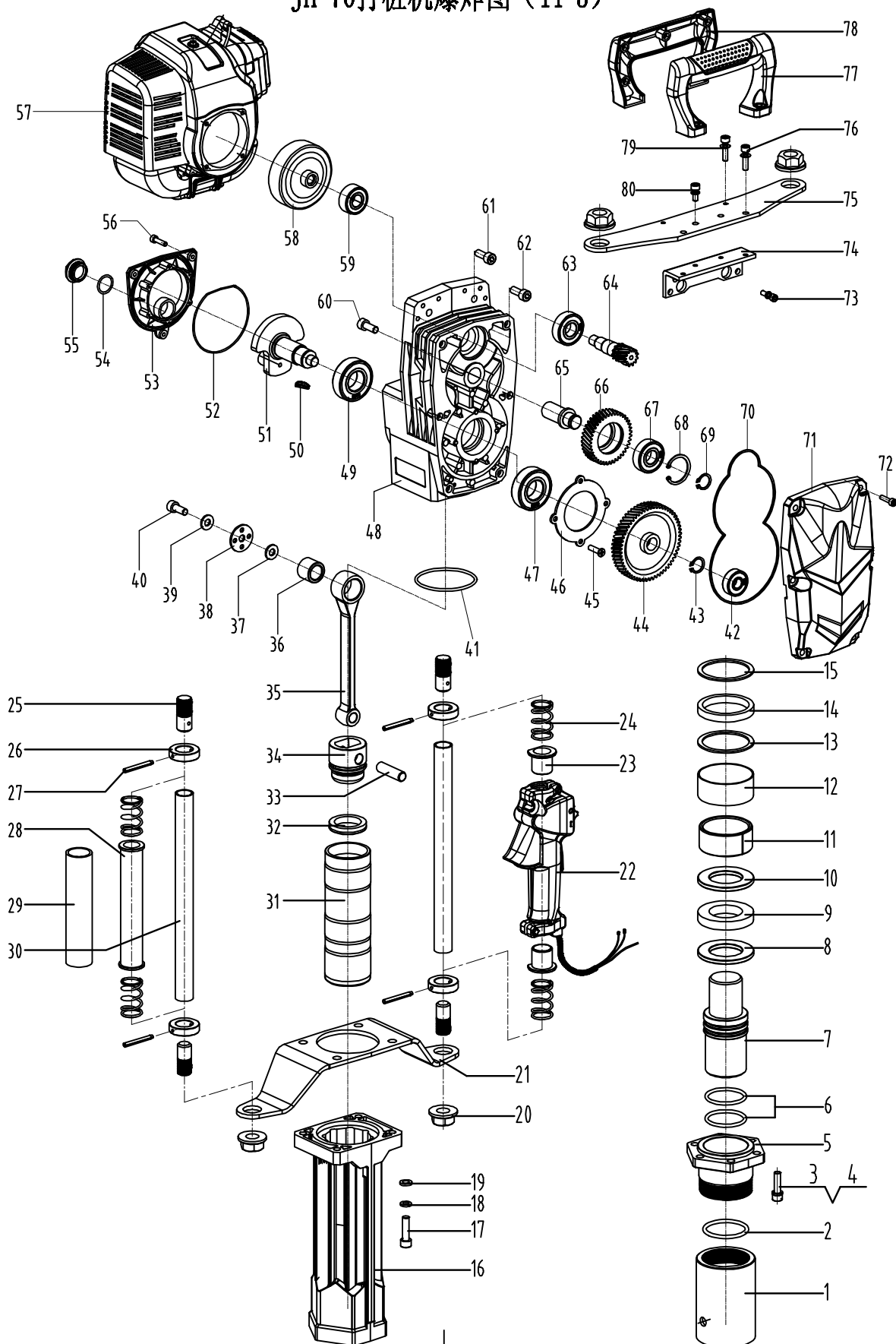
JH-70打桩机爆炸图 (44-5)
