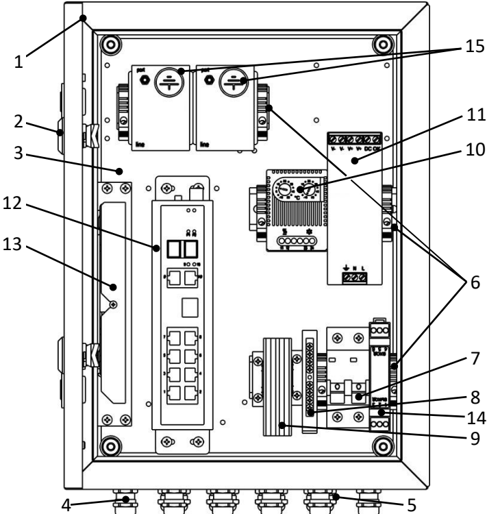
Рисунок 1 – Устройство шкафа
