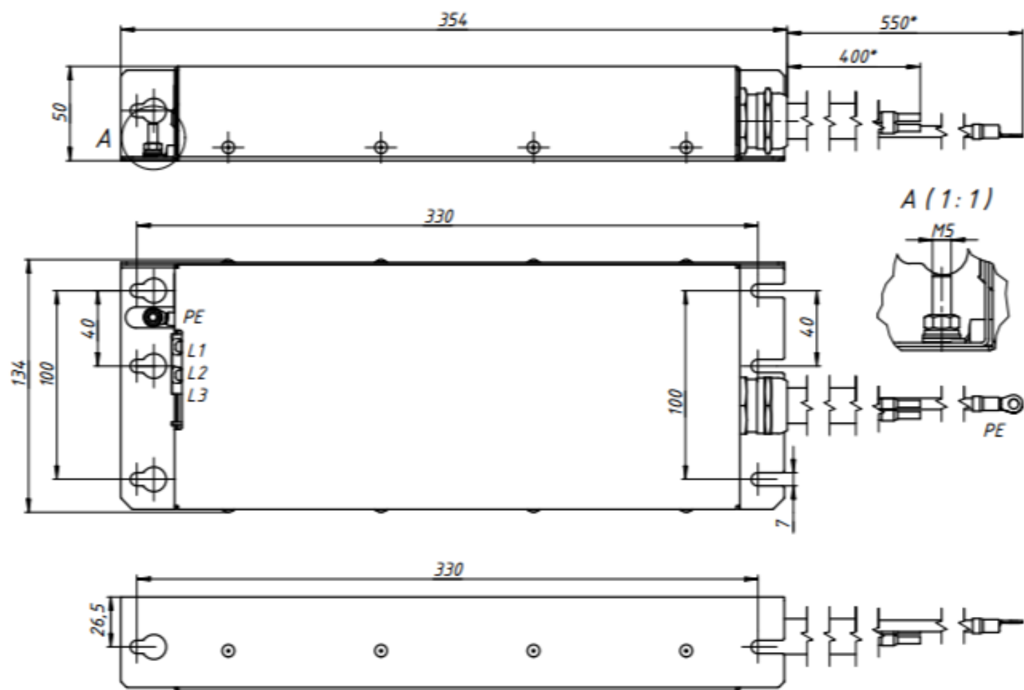
Габариты и присоединительные размеры фильтров ФКРС-5,5(7,5-11)-04-01
