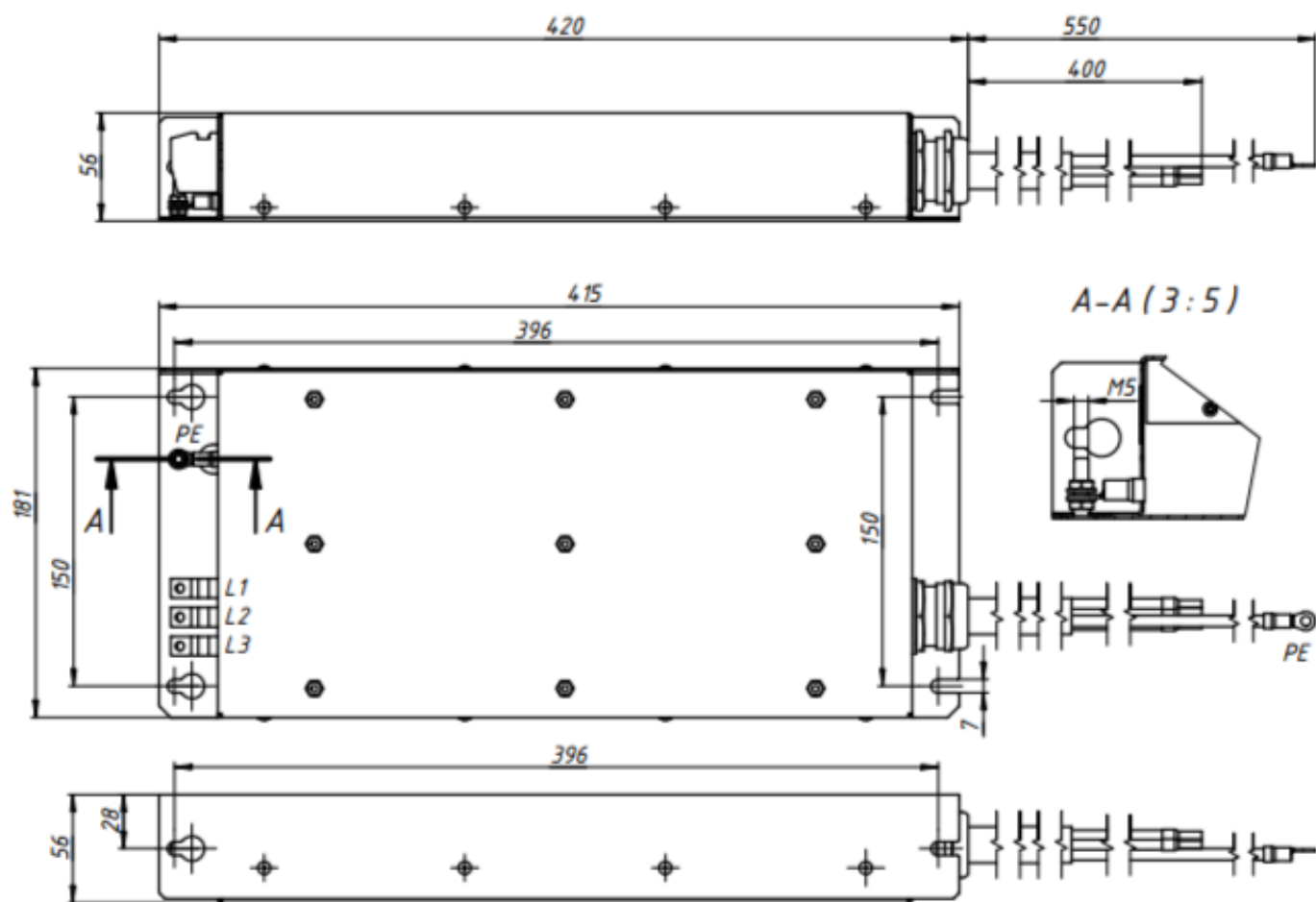
Габаритные и присоединительные размеры ФКРС-15(18,5-22)-0,4-01
