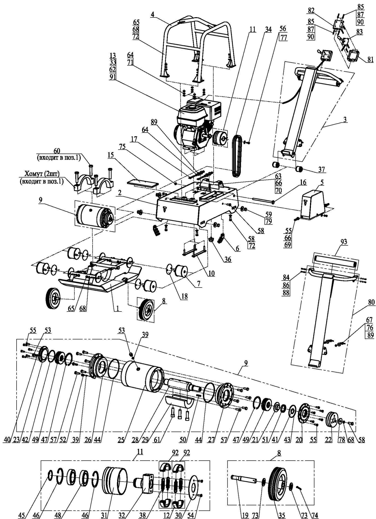
Рисунок 10 – Компоновка виброплиты
