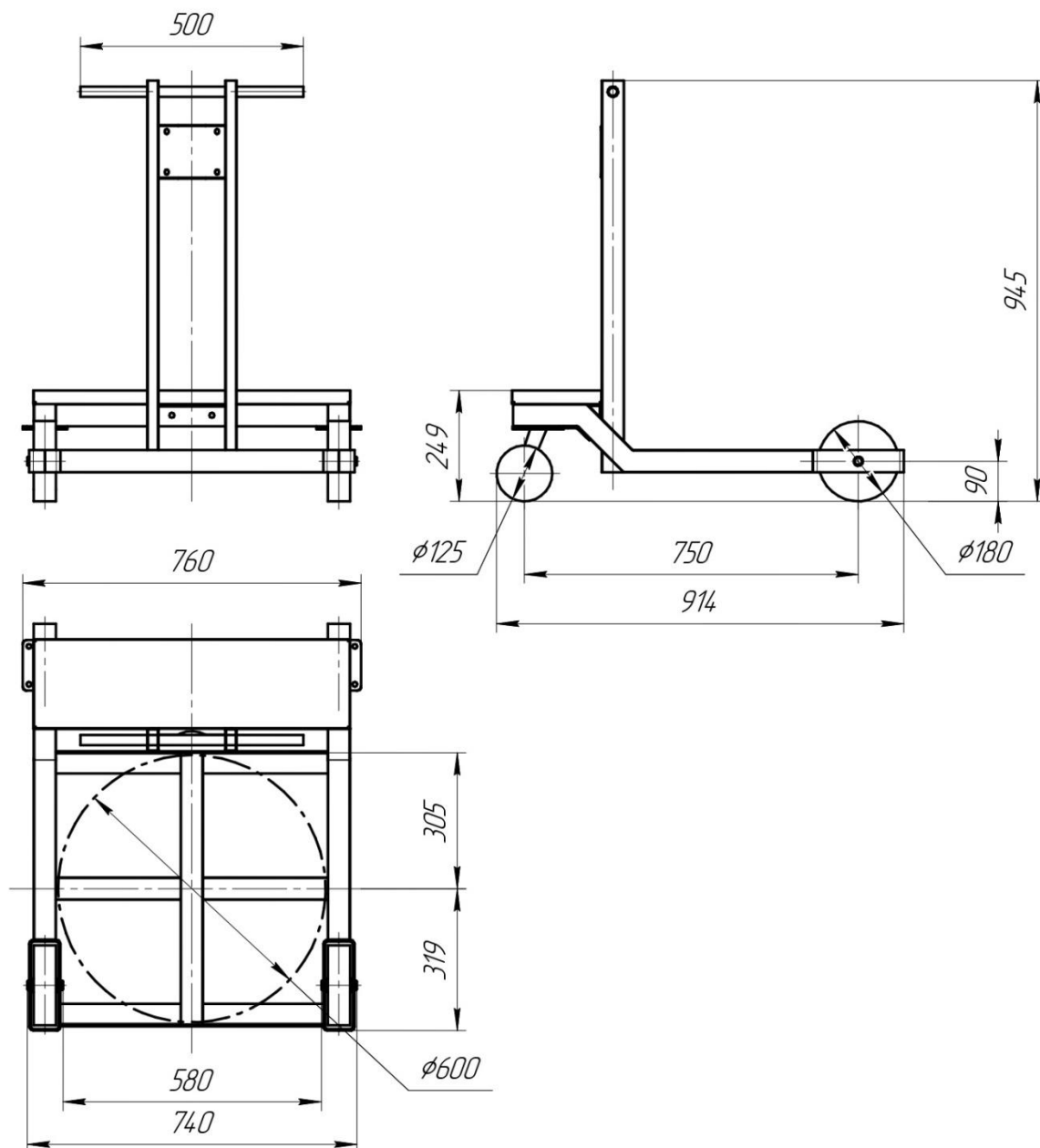
Рисунок 2. Габаритные размеры.
