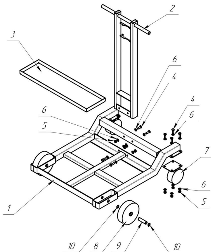
Рисунок 3. Состав тележки.
