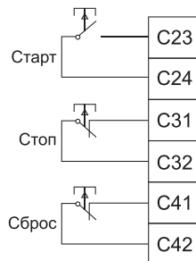
Четырёхпроводное управление
