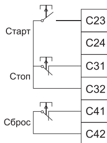
Трёхпроводное управление
