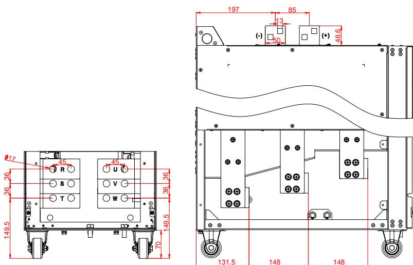
Рис. 4-30 Клеммы силовых цепей 3ф 380В 280–355 кВт стандартные модели и модели (-L1) со встроенными реакторами постоянного тока (единица измерения: мм)
