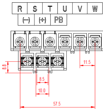
Рис. 4-20 Клеммы силовых цепей 3ф 380В 1,5–7,5 кВт (единица измерения: мм)
