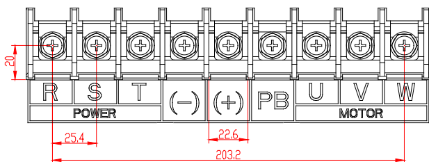
Рис. 4-23 Клеммы силовых цепей 3ф 380В 55–90кВт (единица измерения: мм)
