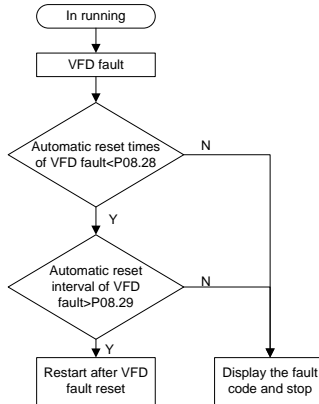
2. Логическая схема запуска после автоматического сброса неисправности
