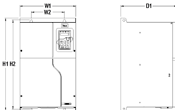
Рис. С-7 Чертеж для настенного монтажа моделей ПЧ 380В 110–132кВт
