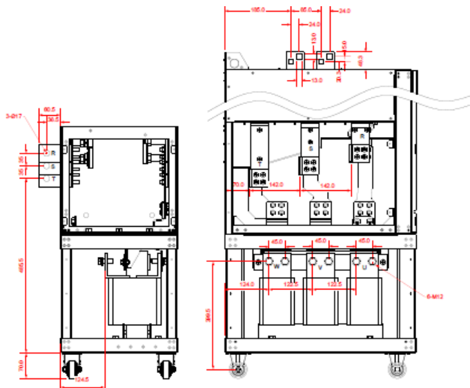
Рис. 4-31 Клеммы силовых цепей 3ф 380В 280–355Вт (-L3) модели с выходными реакторами (единица измерения: мм)
