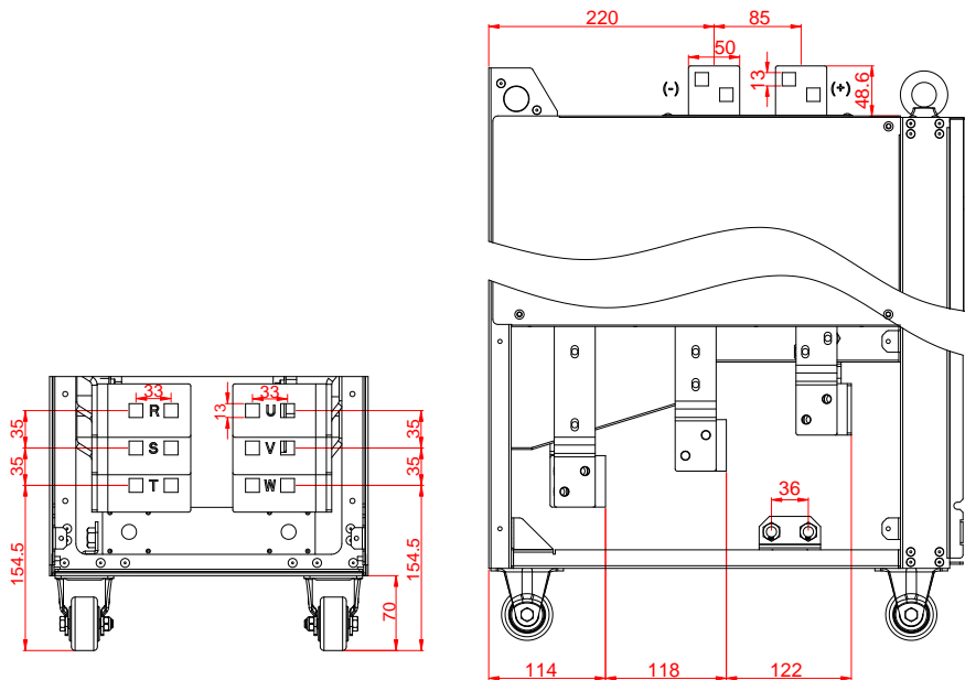
Рис. 4-268 Клеммы силовых цепей 3ф 380В 220–250кВт стандартные модели и модели (-L1) со встроенными реакторами постоянного тока (единица измерения: мм)
