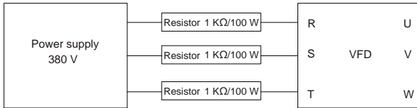
Рис. 8-2 Пример схемы зарядки ПЧ 380 В
