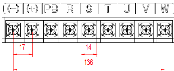
Рис. 4-22 Клеммы силовых цепей 3ф 380В 18,5–22 кВт (единица измерения: мм)
