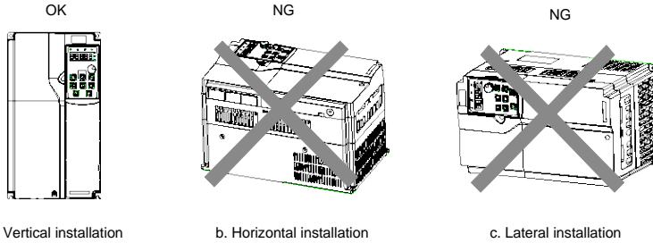
Рис. 4-1 Направление установки ПЧ
