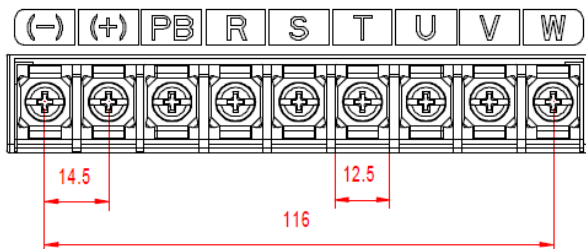
Рис. 4-21 Клеммы силовых цепей 3ф 380В 11–15 кВт (единица измерения: мм)
