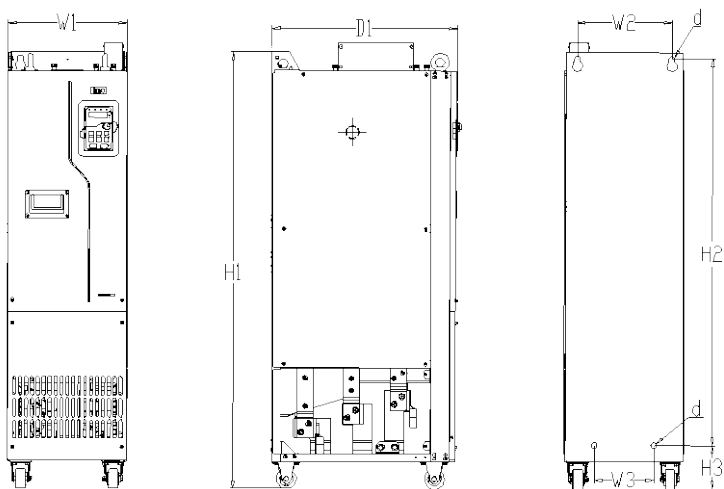
Рис. С-9 Чертеж для настенного монтажа моделей ПЧ 380В 220–250кВт
