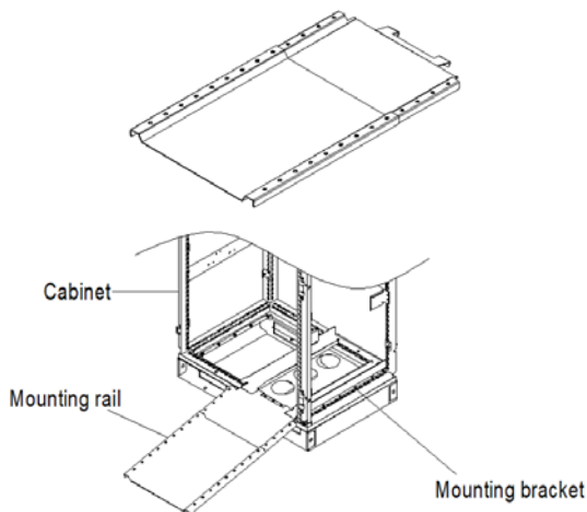
Рис. 4–14 Схема установки монтажной платформы
