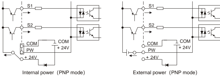
Рис. 4–32 PNP режим
