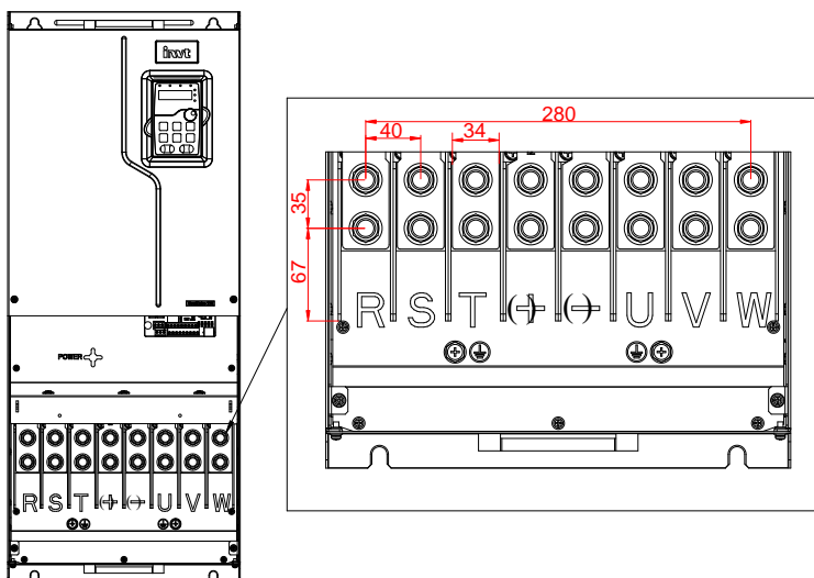
Рис. 4-257 Клеммы силовых цепей 3ф 380В 160–200кВт (единица измерения: мм)
