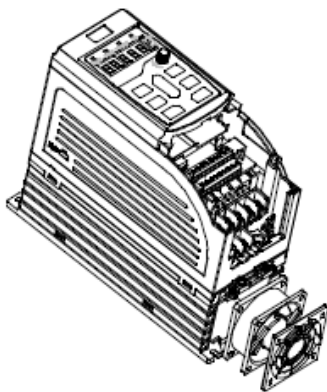
Рис. 8–1 Обслуживание вентиляторов для моделей ПЧ 1.5кВт–7.5кВт
