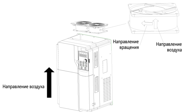
Рис. 8-2 Обслуживание вентиляторов для моделей ПЧ 11кВт–200кВт
