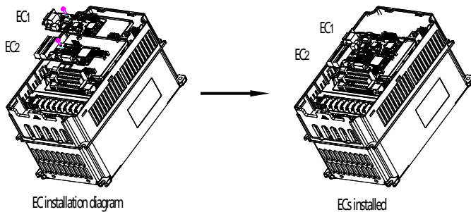
Рис А.2 ПЧ 11кВт – 500 кВт с установленными платами расширения
