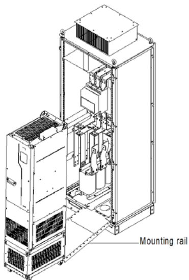
Рис. 4–14 Схема установки монтажной платформы
