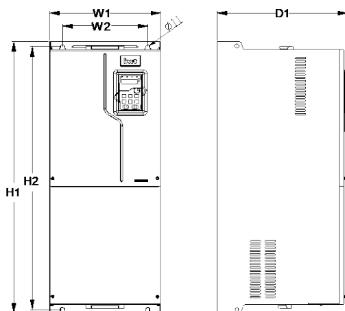
Рис. С-8 Чертеж для настенного монтажа моделей ПЧ 380В 160–200кВт
