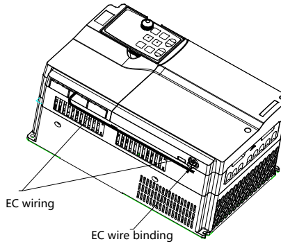
Рис А.6 Прокладка проводов для платы расширения ПЧ от 11 кВт до 500 кВт
