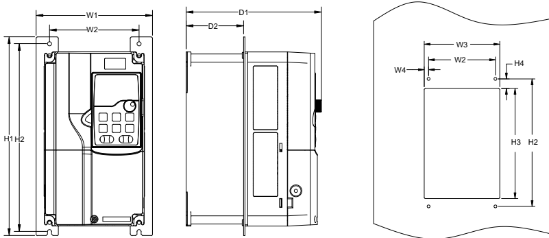
Рис С-12 Чертеж для фланцевого монтажа моделей ПЧ 380 В 30–90кВт
