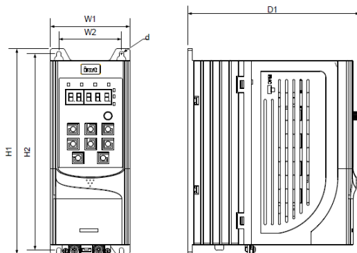
Рис. С-4 Чертеж для настенного монтажа моделей ПЧ 380В от 1,5 до 7,5 кВт
