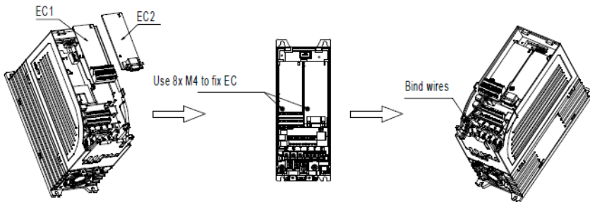
Рис А.1 ПЧ 1,5кВт – 7,5 кВт с установленными платами расширения
