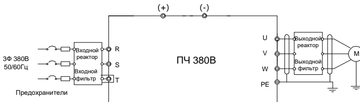
Рис. 4–19 Схема подключения основной цепи AC 3ф 380В
