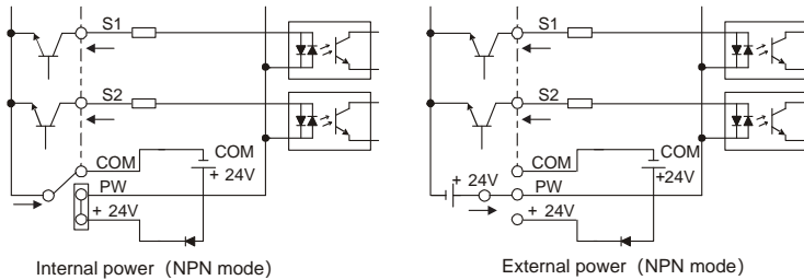
Рис. 4–31 NPN режим
