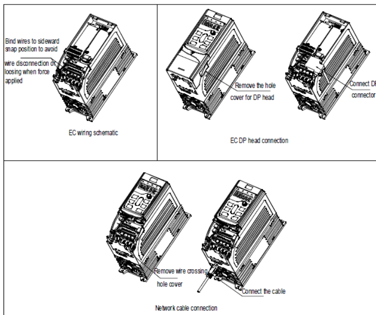
Рис А.5 Прокладка проводов для платы расширения ПЧ от 1,5 кВт до 7,5 кВт
