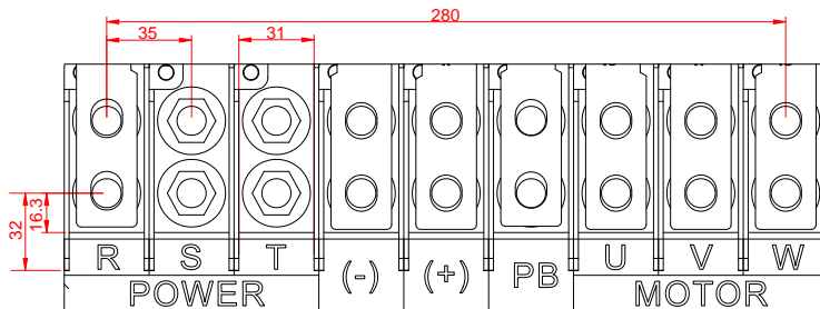
Рис. 4-24 Клеммы силовых цепей 3ф 380В 110–132кВт (единица измерения: мм)
