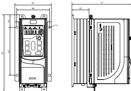
Рис. С-10 Схема фланцевого монтажа ПЧ напряжением 380 В, от 1,5 до 7,5 кВт
