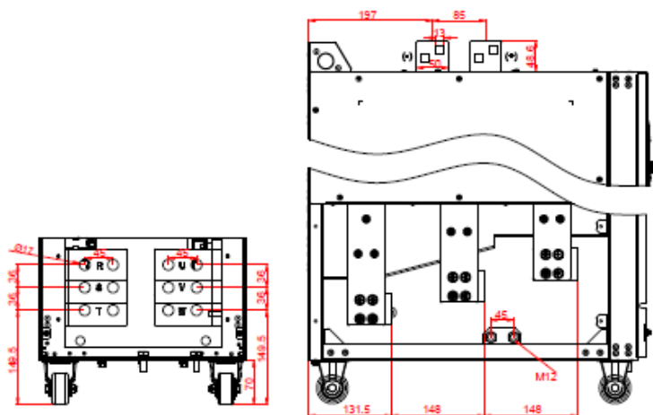
Рис. 4-31 Клеммы силовых цепей 3ф 380В 280–355Вт (-L3) модели с выходными реакторами (единица измерения: мм)
