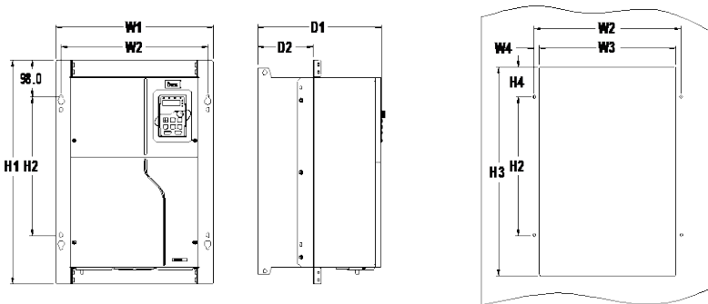
Рис. С–13 Чертеж для фланцевого монтажа моделей ПЧ 380В110-200кВт
