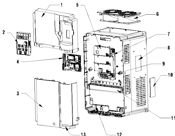
Рис. 3-5 Конструкция ПЧ
