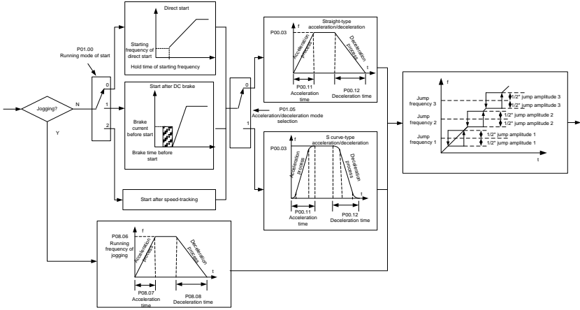
1. Логическая схема для запуска после перезапуска при отключении питания
