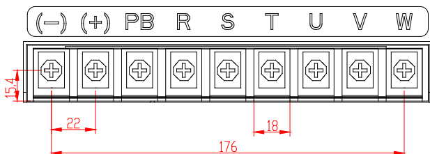
Рис. 4-24 Клеммы силовых цепей 3ф 380В 45кВт (единица измерения: мм)
