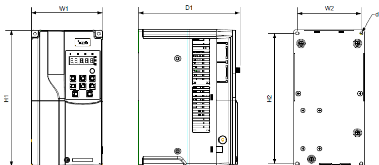
Рис С.1 Чертеж для настенного монтажа моделей ПЧ 380В, от 11 до 45 кВт
