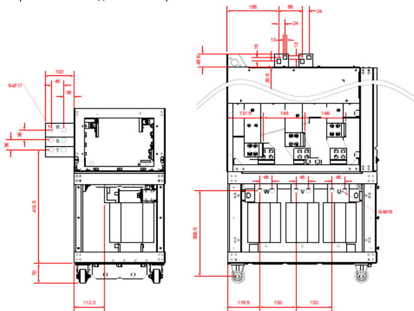
Рис. 4-33 Клеммы силовых цепей 3ф 380В 400–500 кВт (-L3) модели с выходными реакторами (единица измерения: мм)
