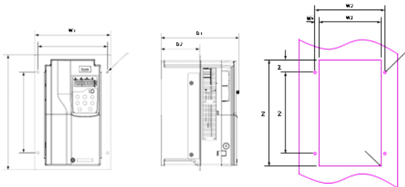
Рис С-2 Схема фланцевого монтажа ПЧ напряжением 380 В, от 11 до 22 кВт
