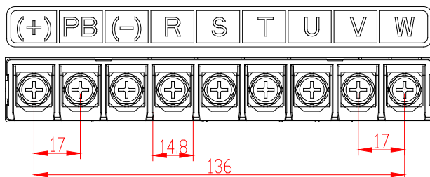
Рис. 4-22 Клеммы силовых цепей 3ф 380В 30–37кВт (единица измерения: мм)
