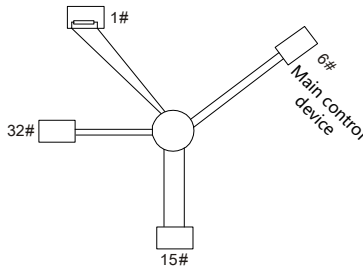
Рис. 9–5 Подключение «Звезда»
