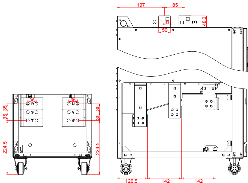
Рис. 4-279 Клеммы силовых цепей 3ф 380В 280–355кВт (-L3) модели с выходными реакторами (единица измерения: мм)
