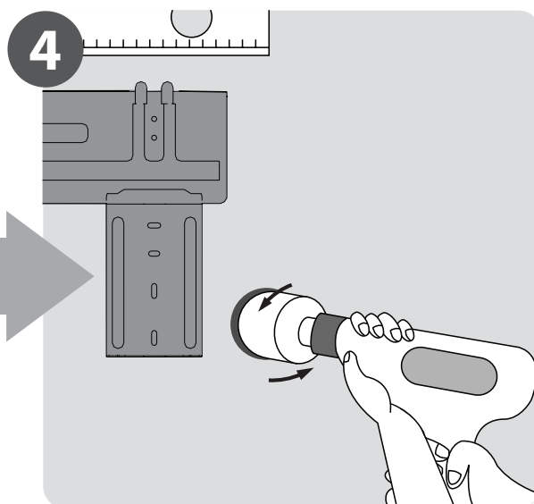
Сверление отверстия в стене (Стр. 10)
