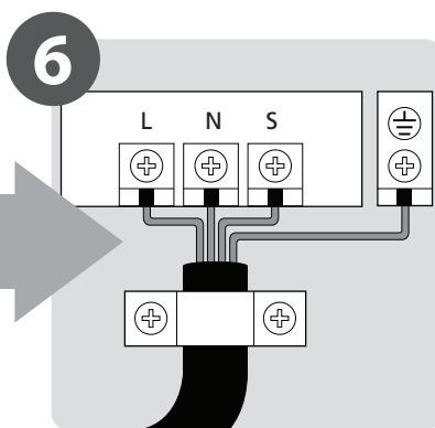
Подсоединение проводки (Стр. 15)
