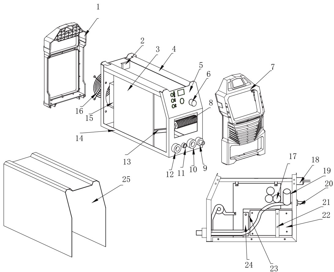
Схема сборки № 1
