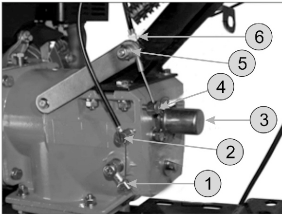
Рис. 5 Подключение тросов управления
