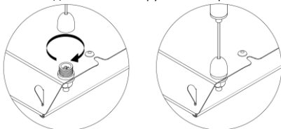
Рисунок 7 — Подвесной монтаж.
