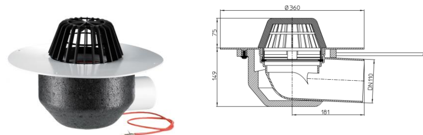
Рис. 2. Кровельная воронка HL64.1P/1.
